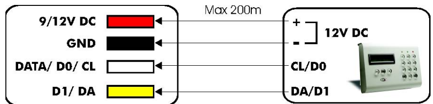
Fig. 3 - = Esempio Connessione Wiegand / Clock &amp; Data
