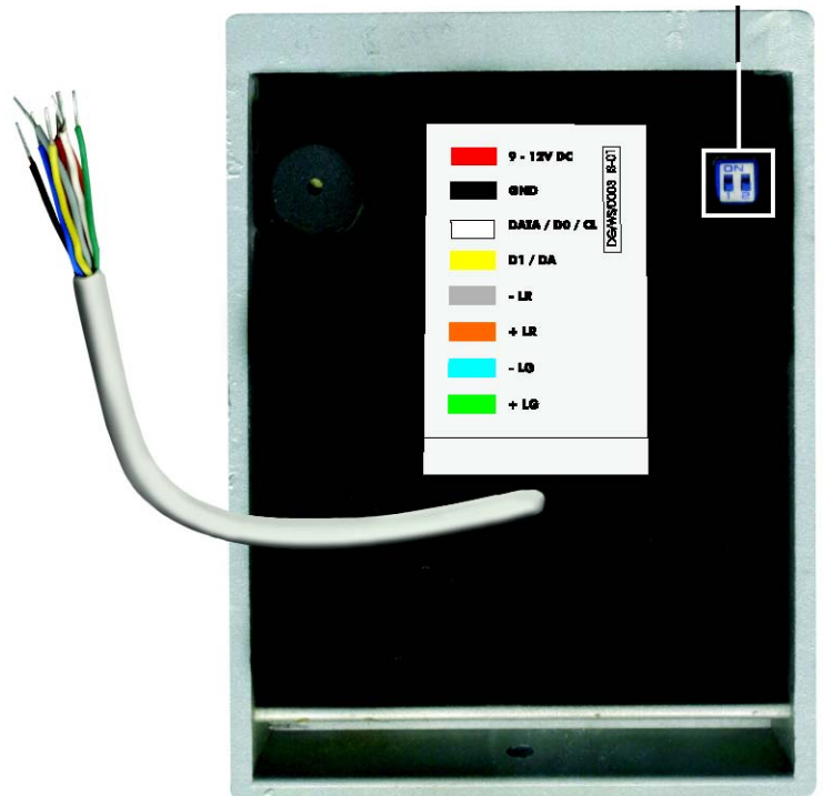
Fig. 2 - VKP : Vista Retro
